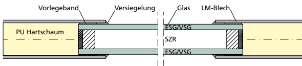
Schematische Darstellung eines Türelementes
