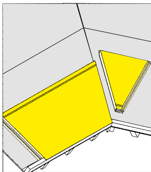
3. ... Plattenhauptstück in die Kehle legen (die Überlappung liegt auf der Traufbohle), Reststück drehen ...
